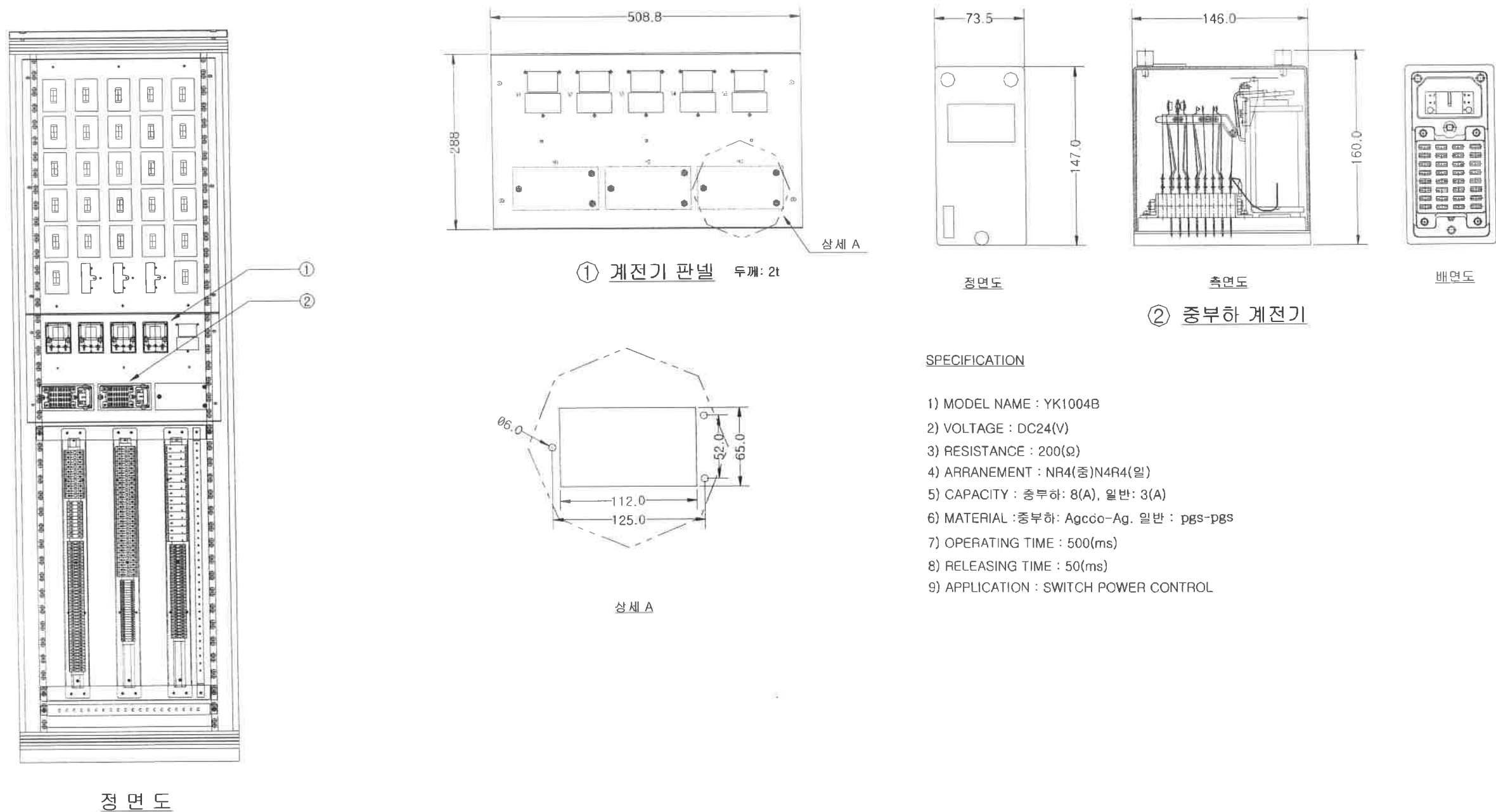
그림 3. 계전기 판넬 (중부하계전기)
