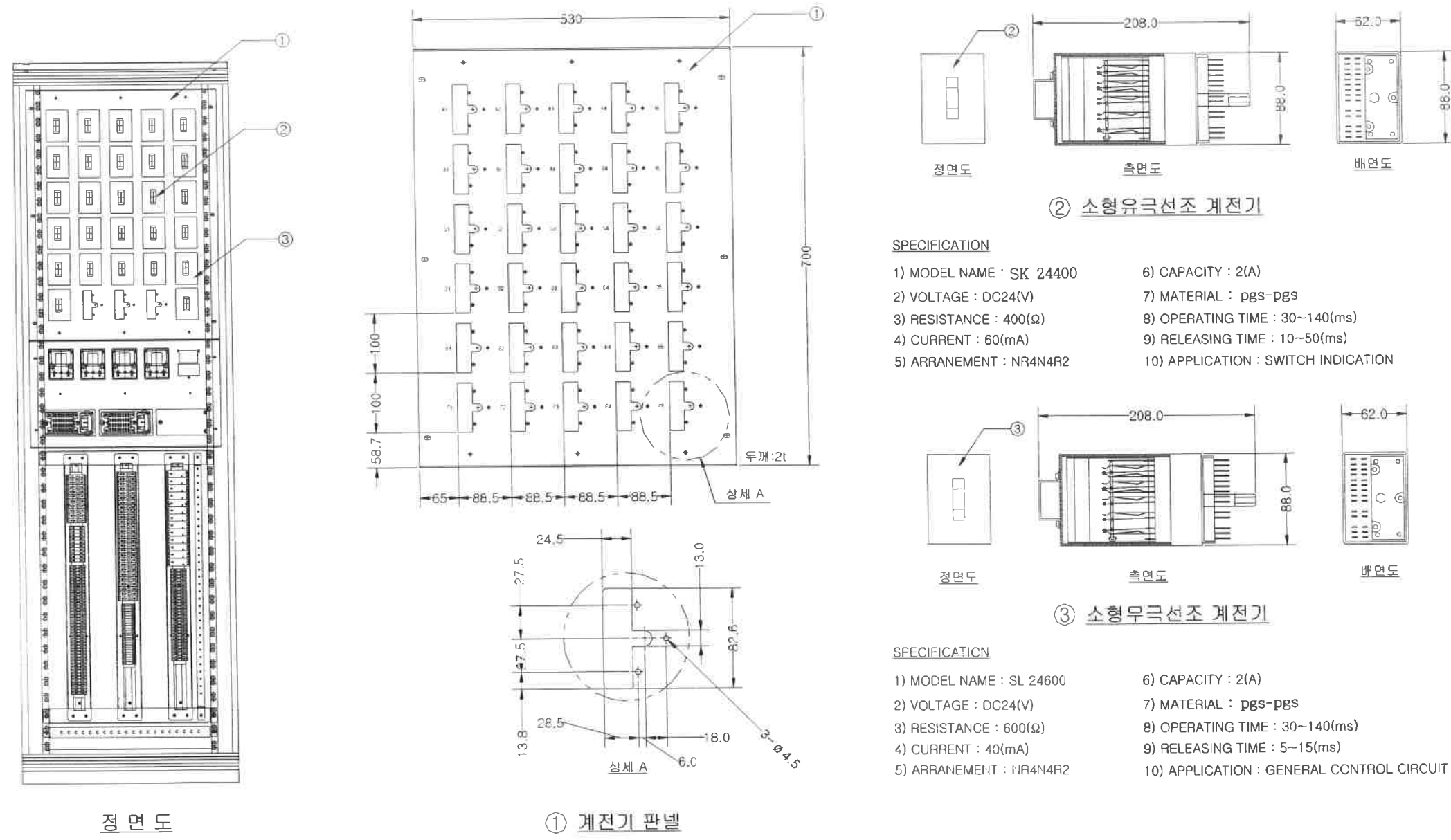
그림 2. 계전기 판넬 (소형무극, 소형유극선조 계전기)
