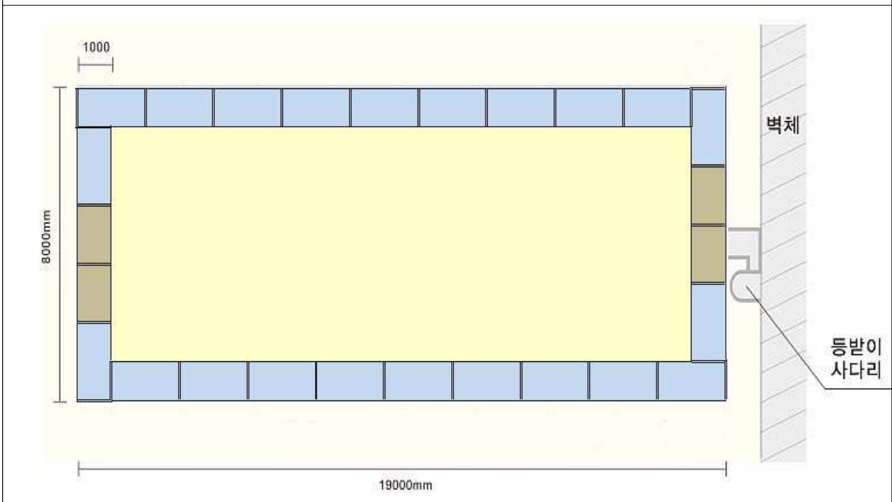
달대형 점검로 도면
