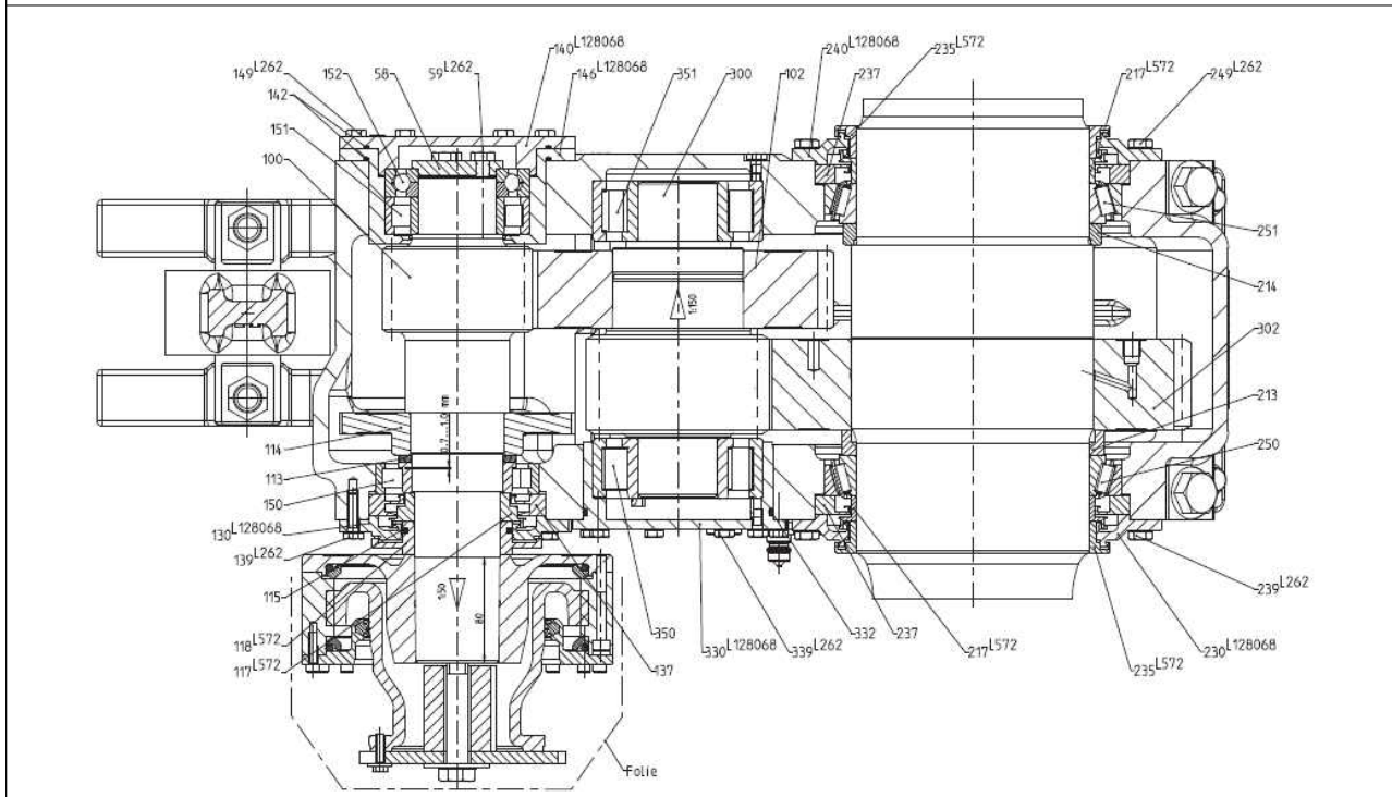
구동기어 도면
