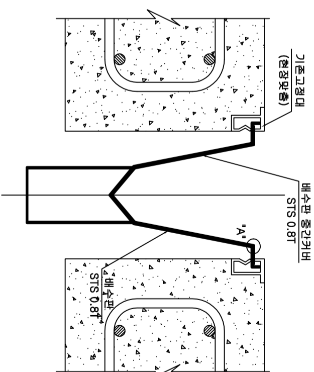
단면도 (중앙부)
